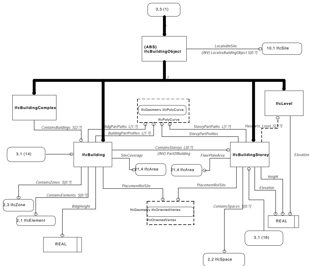
図8 Express-G ダイアグラムの例
